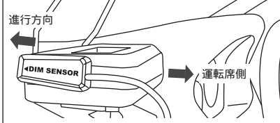
【図4-2】DIMセンサーの取付方向
