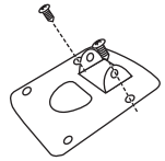
【図4-1】DIMセンサーを固定する
